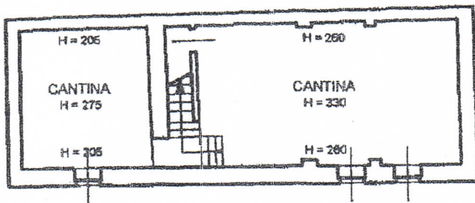
PIANTA PIANO INTERRATO
